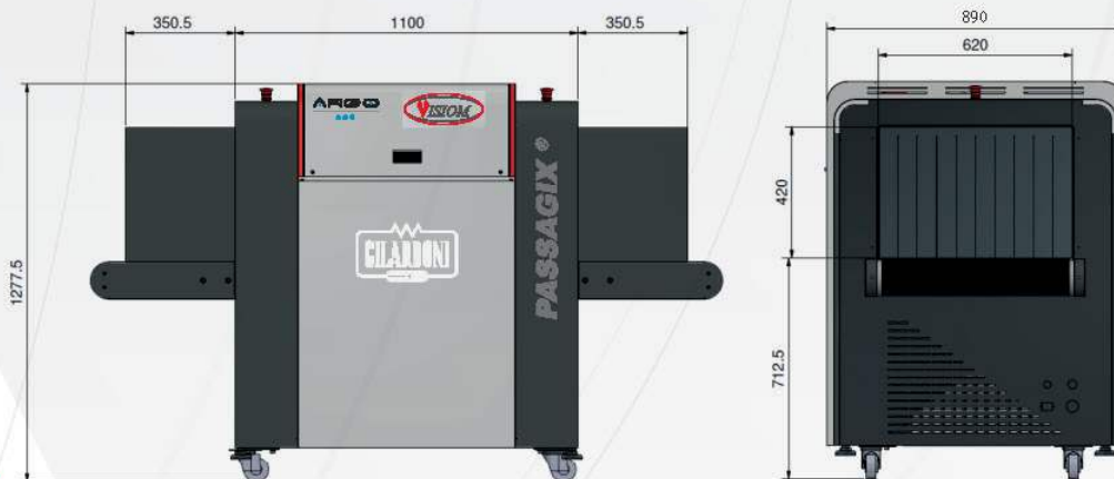
Dimensions en mm
